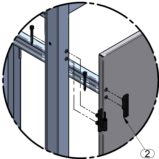
DETAIL A TYP 3 Places
